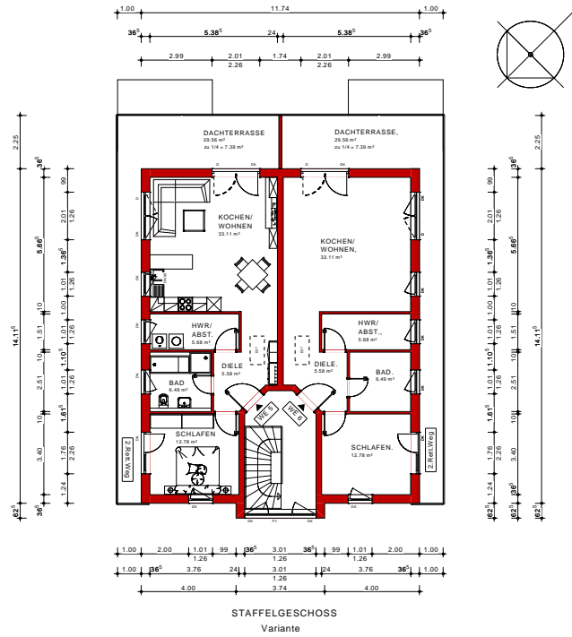
GRUNDRISS
